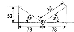
Schema angolarità crocette Crocetta superiore lunghezza cm. 55 da centro Crocetta inferiore lunghezza cm. 89 da centro
