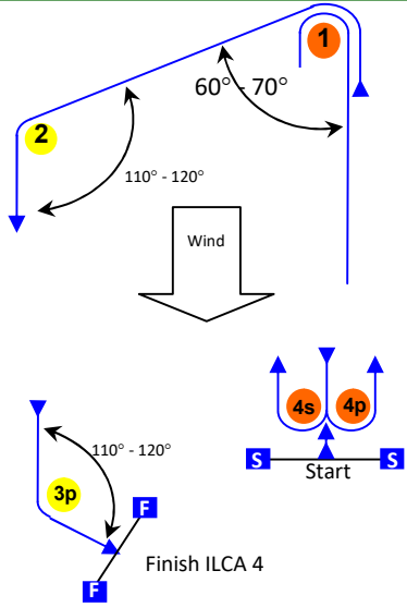
ILCA 4 START -1 – 4S/4P -1 - -2 – 3p - FINISH
