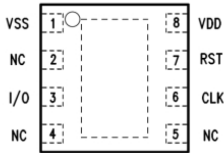
图 22 C2×2eSIM 芯片管脚示意 (TOP VIEW)
